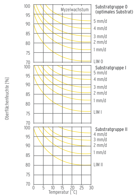
Bild B: Verallgemeinertes Isoplethensystem für das Myzelwachstum, das für alle in Bauteilen auftretenden Pilze gilt (nach Sedlbauer 2001); Bild oben gilt für optimales Substrat, Mitte für Substratgruppe I und Bild unten für Substratgruppe II. Die angegebenen Werte in mm/d charakterisieren das zu erwartende Wachstum. LIM bedeutet: Lowest Isopleth for Mould = unterste Wachstumsgrenze
