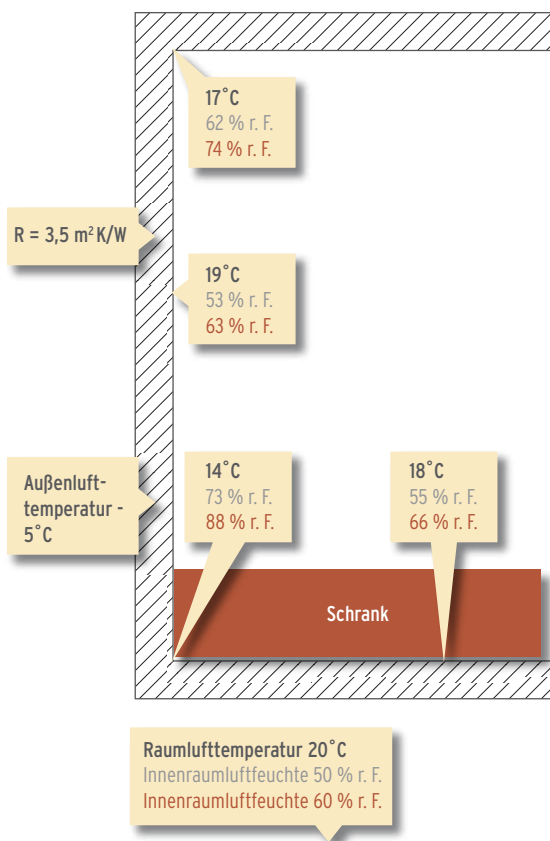
Bild 5: Darstellung der Auswirkung von Außenecken (Wärmebrücken) und Möblierungen auf die Wandtemperatur und die relative Feuchte an der Oberfläche (Oberflächenfeuchte) der Innenwand, bei zwei ausgewählten Raumlufffeuchten (50 % und 60 %). Durch den vorgebauten Schrank wird die Wandtemperatur in diesem Bereich nochmals gegenüber der nicht verstellten Raumecke erniedrigt.
