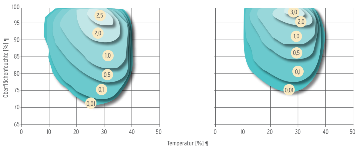
Bild 2: Isoplethensysteme für Myzelwachstum der Schimmelpilze Aspergillus restrictus (links) und Aspergillus versicolor (rechts) in Abhängigkeit von relativer Oberflächenfeuchte und Temperatur nach Smith et al. (1982). Die Zahlen an den Isoplethen kennzeichnen die Wachstumsraten in Millimeter pro Tag (mm/d).
