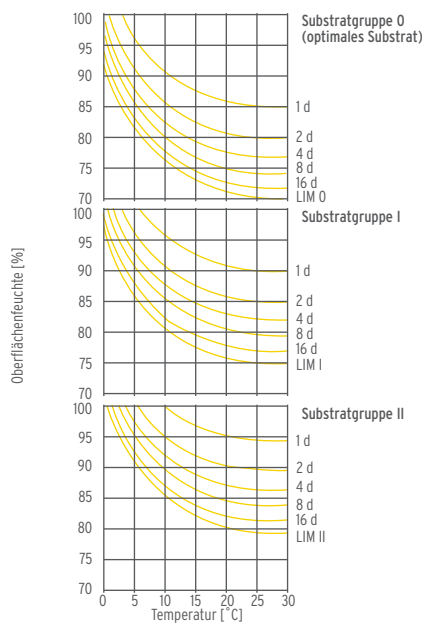
Bild A: Verallgemeinertes Isoplethensystem für die Sporenauskeimung, das für alle in Bauteilen auftretenden Pilze gilt (nach Sedlbauer 2001); Bild oben gilt für optimales Substrat, Mitte für Substratgruppe I und Bild unten für Substratgruppe II. Die angegebenen Werte charakterisieren die Zeitdauer, nach welcher eine Keimung abgeschlossen ist. LIM = Lowest Isopleth for Mould = unterste Grenze der Sporenauskeimung
