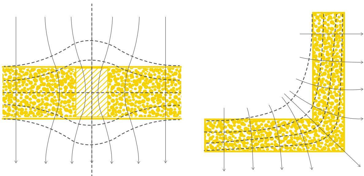
Bild 4: Schematische Darstellung zweier Wärmebrücken mit Angabe der Wärmeströme (Adiabaten; durchgezogene Linien) und Isothermen (gestrichelte Linien). Wärmebrücken zeichnen sich physikalisch durch verstärkten Wärmefluss mit Verdichtung der Adiabaten und Wölbung der Isothermen aus (nach Gertis et al. 2001)
