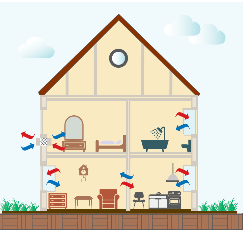
Bild 12: Ventilatorgestützte Lüftung: Dezentrales Lüftungsgerät (rot = Abluft; blau = Zuluft)
