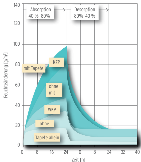
Bild 8: Wasserdampfabsorption von Kalkzementputz (KZP) und Weißkalkputz (WKP) ohne und mit Raufasertapete sowie von der Tapete allein (aufgeklebt auf Metallplatte) bei Änderung der relativen Luftfeuchte von 40 % und 80 % und anschließende Desorption bei Absenken der Luftfeuchte von 80 % auf 40 % (Messung an Proben im Klimaraum)
