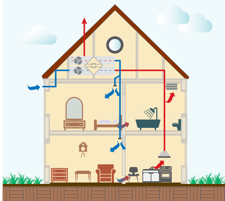
Bild 11: Ventilatorgestützte Lüftung: Zu- und Abluftanlagen (rot = Abluft; blau = Zuluft)
