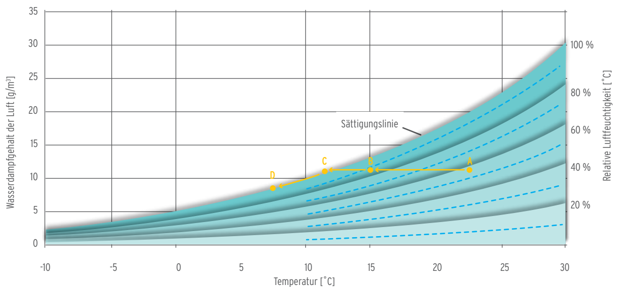
Bild 3: Wasserdampfgehalte der Luft in Abhängigkeit von Raumlufttemperatur und relativer Luftfeuchte. Weitere Erläuterungen im Text.
