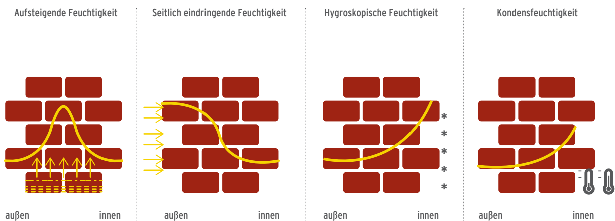
Bild 15: Feuchtigkeitsprofile in der Wand
